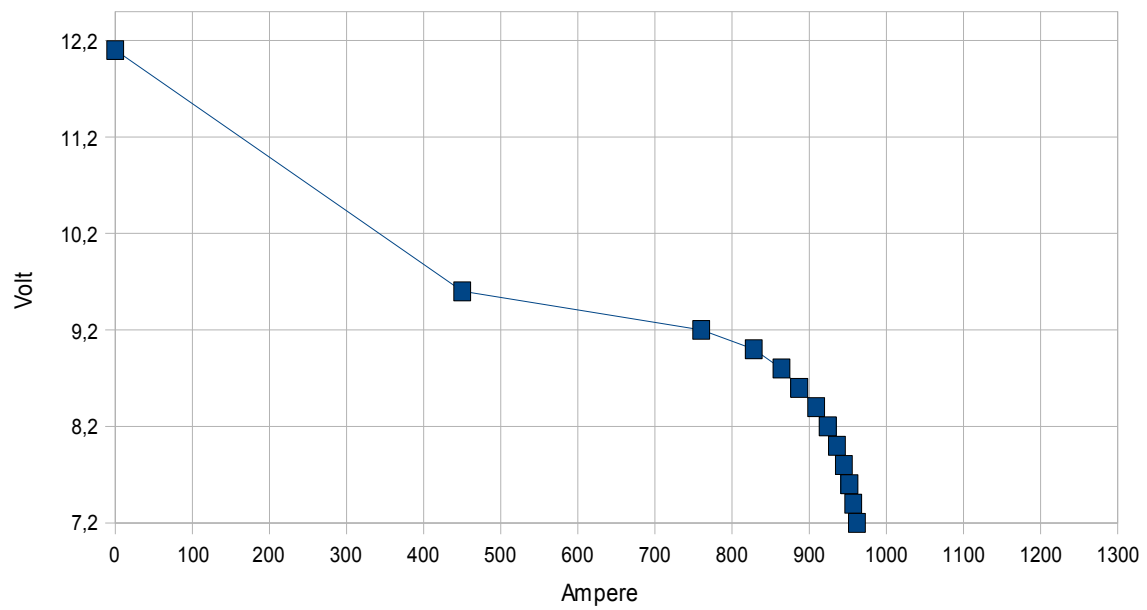
Entladediagramm
